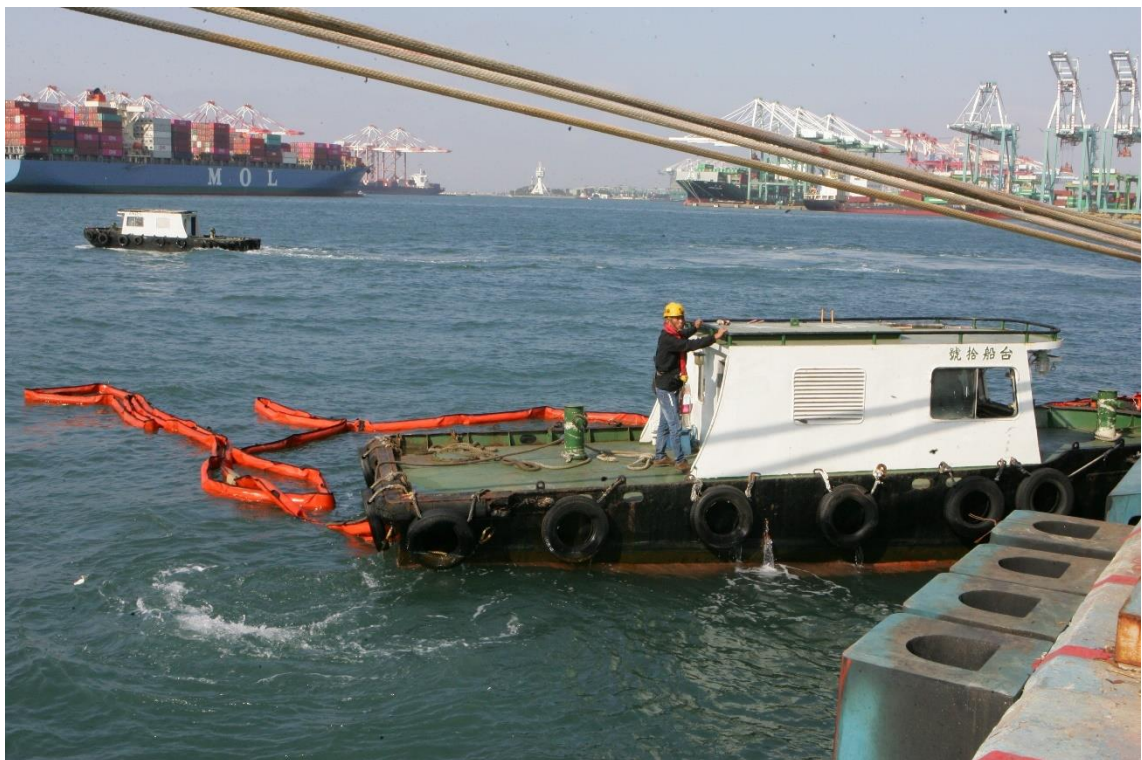
海域佈設第二道攔油索
